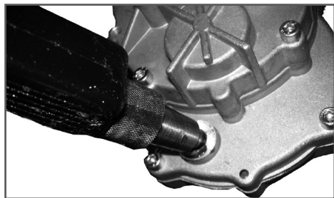
Рис. 15 Обслуживание редуктора
